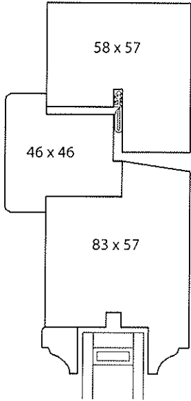
coupe verticale
